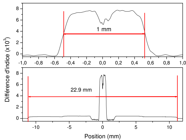
Figure 2.7 - Préforme H1
