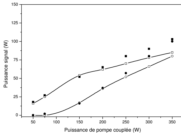
Figure 2.67 – Comparaison entre les mesures d'ORC ([2.42]) à 1.5 \mu\text{m} (■) et 1 \mu\text{m} (●) et les résultats de modélisation en appliquant le modèle M5 incluant la variation de température à 1.5 \mu\text{m} (-□-) et à 1 \mu\text{m} (-○-).
