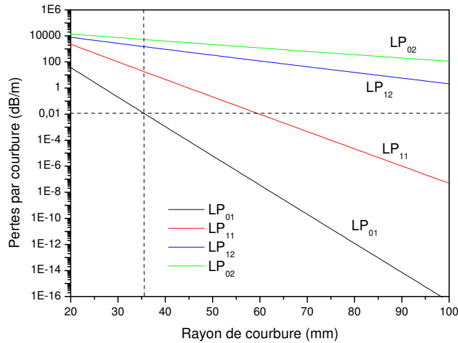
Figure 4.4 – Evolution des pertes par courbure en fonction du rayon de courbure pour une fibre de 30 \mu\text{m} de diamètre et d'ouverture numérique 0,08 à 1,5 \mu\text{m}
