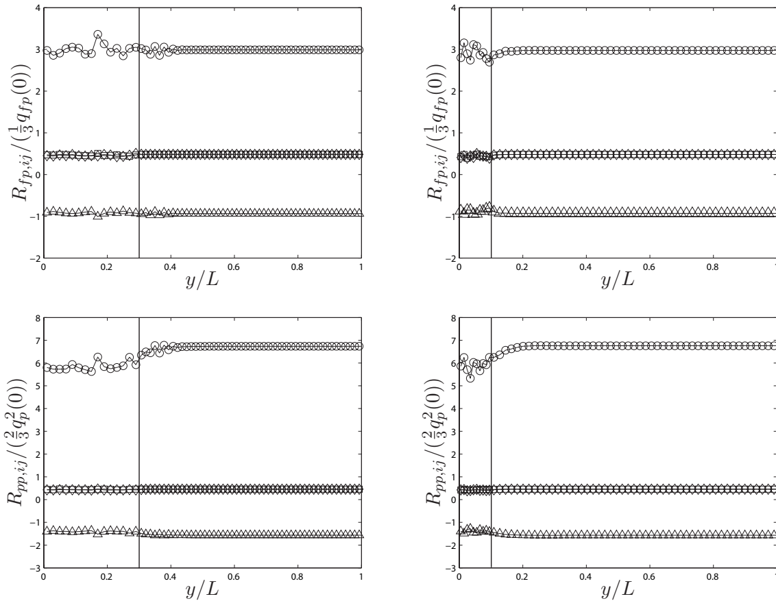
FIG. 5.33 – Profils de contraintes fluide-particules et particulaires à l'instant t = 5/S_f issus de HELM avec \eta = 0,3 (gauche) et \eta = 0,1 (droite); \circ : R_{uu} , \square : R_{vv} , \diamond : R_{ww} , \triangle : R_{uv} .
