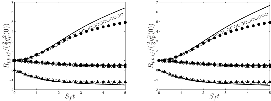
FIG. 5.31 – Développements des contraintes particulières prédits par HELM avec \eta = 0,3 (gauche) et \eta = 0,1 (droite). \circ : moyenne dans le domaine lagrangien ( \circ : R_{pp,uu} , \langle R_{pp,uu} \rangle^- , \square : R_{pp,vv} , \langle R_{pp,vv} \rangle^- , \diamond : R_{pp,ww} , \langle R_{pp,ww} \rangle^- , \triangle : R_{pp,uv} , \langle R_{pp,uv} \rangle^- ); — : moments au 5ième point du maillage pression eulérien ; \bullet : LES/DPS (Laviéville [1997]).
