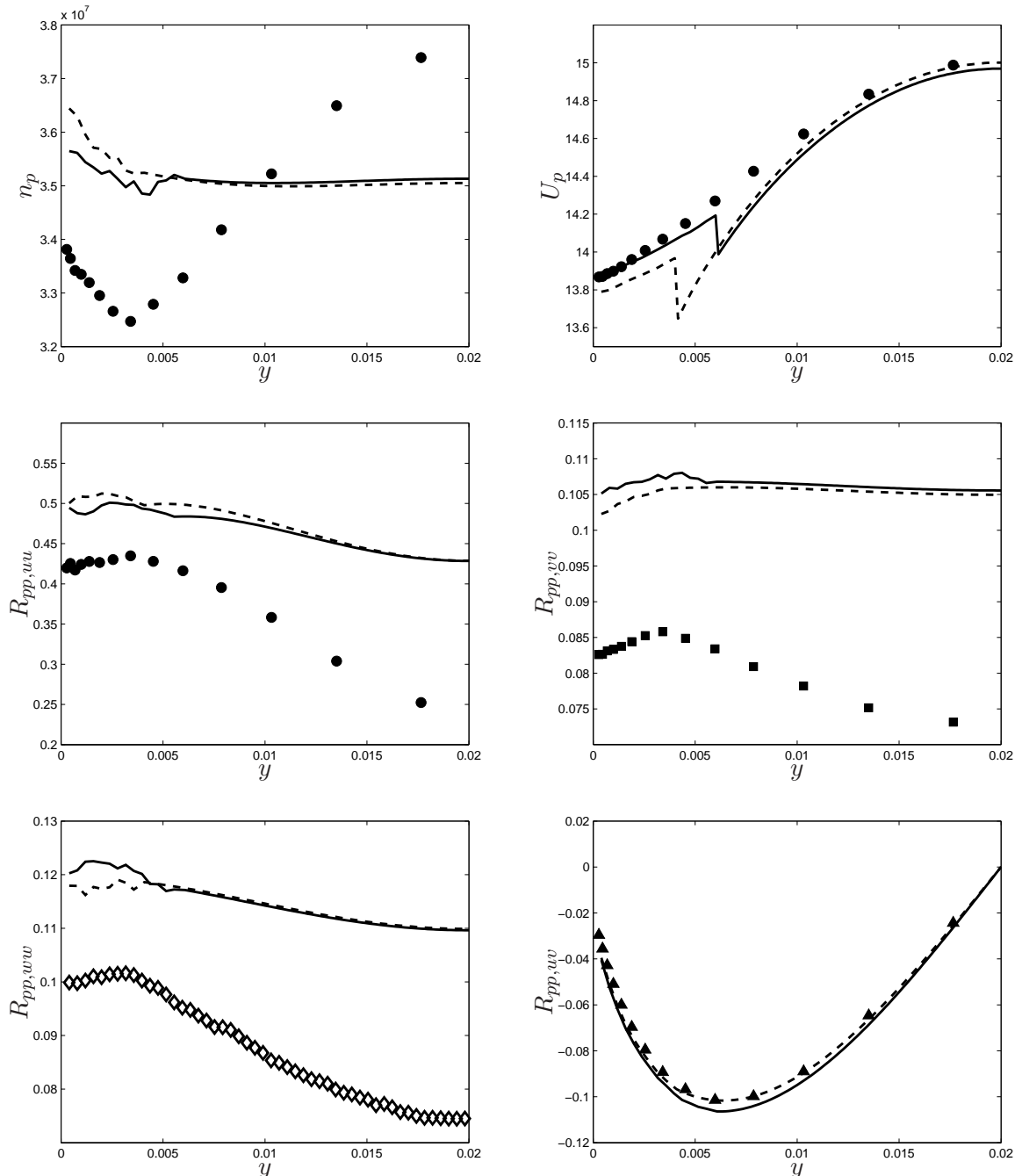
FIG. 6.19 – Influence du rapport de volume \eta dans le cas B3. \circ : lagrangien stochastique ; - \cdot - \cdot - : eulérien (6.19) ; — : HELM avec \eta = 0, 3 ; \cdots \cdots : HELM avec \eta = 0, 2 ; \bullet : DPS (Sakiz [1999]).
