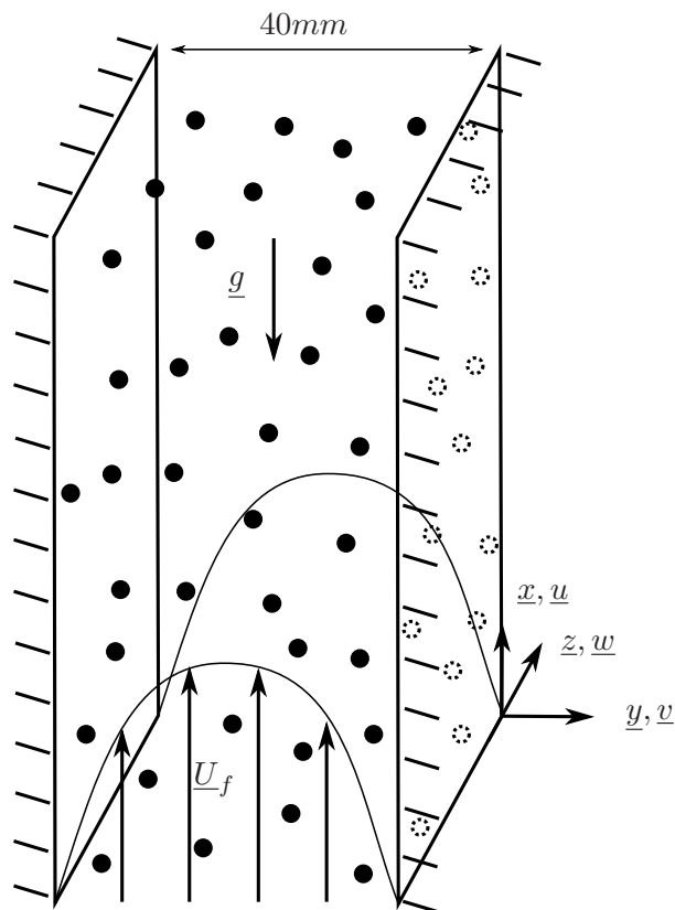
FIG. 6.1 – Description de l'écoulement test.
