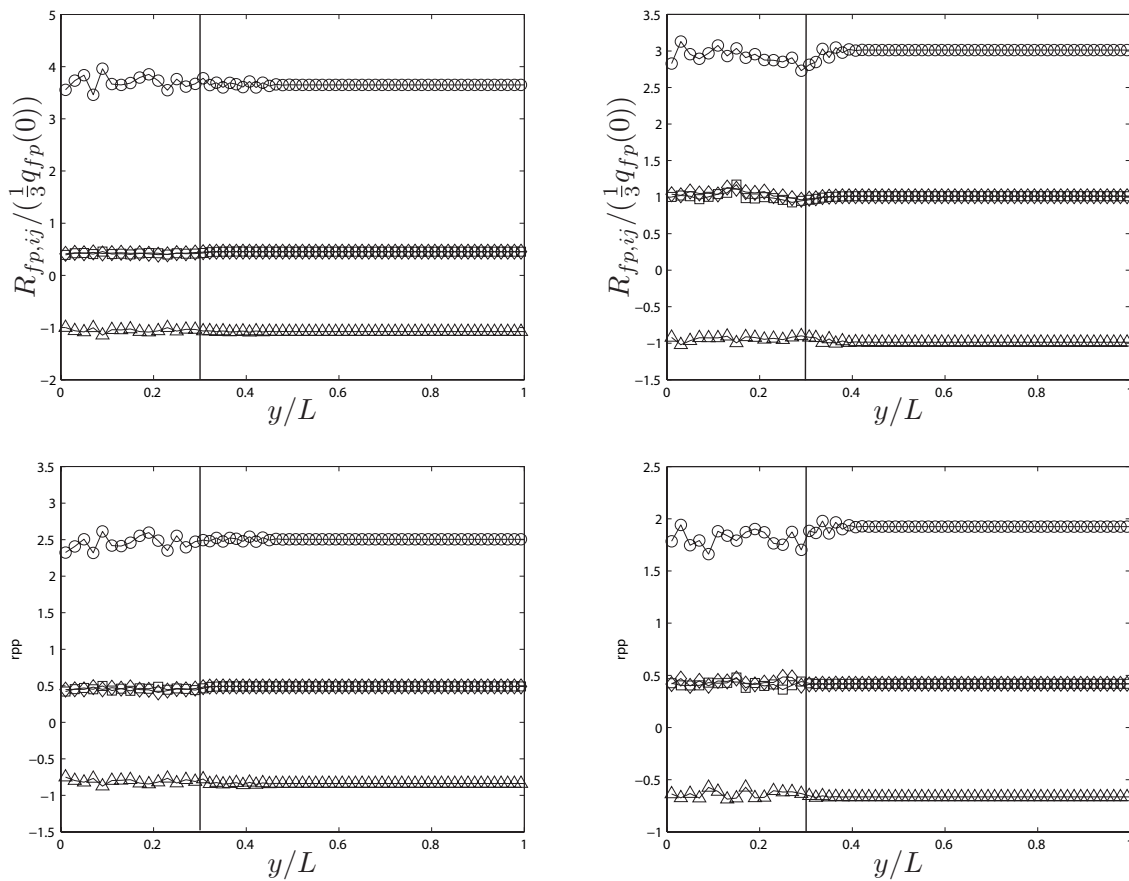
FIG. 5.36 – Profils de contraintes fluide-particules et particulaires à l’instant t = 5/S_f issus de HELM avec \eta = 0, 3 pour le cas B (gauche) et le cas Ac (droite); \circ : R_{uu} , \square : R_{vv} , \diamond : R_{ww} , \triangle : R_{uv} .
