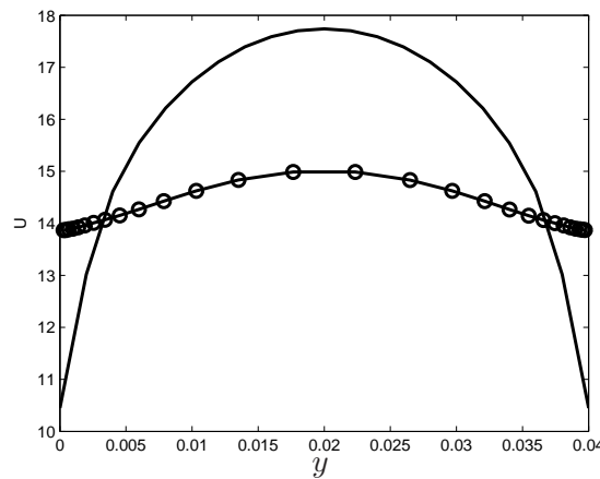
FIG. 6.2 – Profils de vitesse moyenne longitudinale du fluide (—) et de vitesse moyenne des particules dans le cas B3 (—○—).
