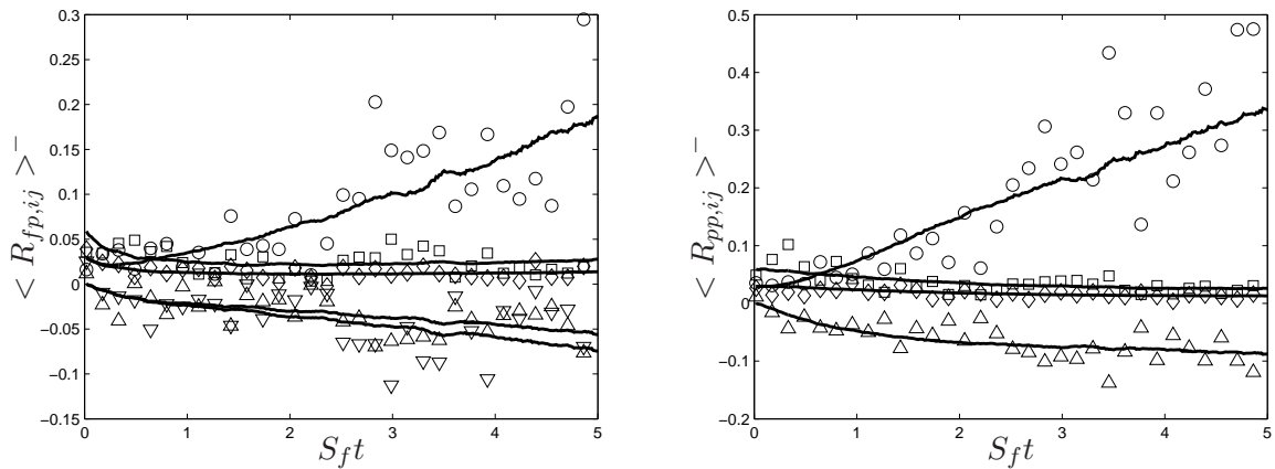
FIG. 5.22 – Développements des contraintes fluide-particules entrantes (gauche) et des contraintes particulières entrantes (droite) dans le cas A. \circ : moyennes sur les particules numériques injectées ( \circ : \langle R_{uu} \rangle^- , \square : \langle R_{vv} \rangle^- , \diamond : \langle R_{ww} \rangle^- , \triangle : \langle R_{uv} \rangle^- ); — : moyennes issues de la pdf de Richman associée aux moments eulériens à la face couplage.
