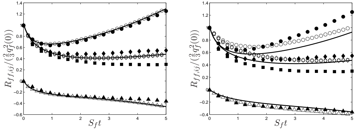
FIG. 5.3 – Développements des contraintes cinétiques du fluide vu par les particules (cas A) prédits par le modèle SLM (gauche) et le modèle LIPM (droite). ; \circ : lagrangien stochastique ( \circ : R_{ff,uu} , \square : R_{ff,vv} , \diamond : R_{ff,ww} , \triangle : R_{ff,uv} ); — : eulérien ; \bullet : LES/DPS (Laviéville [1997]).
