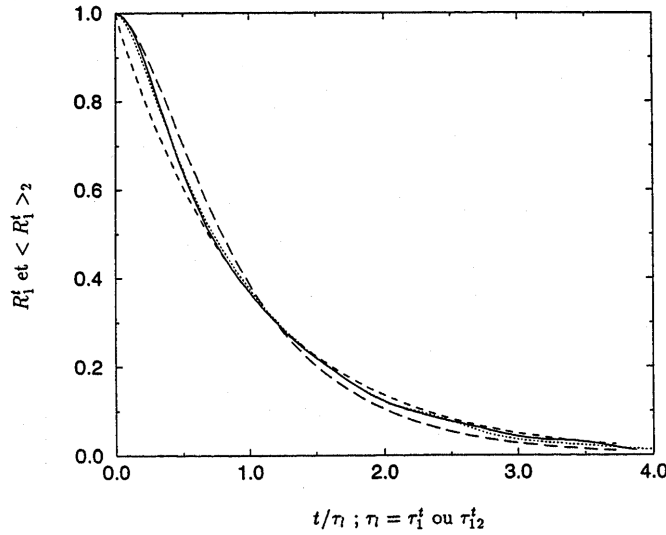
FIG. 1.6 – Fonctions d'autocorrélations temporelles lagrangiennes du fluide R_1^t \equiv \mathcal{R}_f et du fluide "vu" par les particules \langle R_1^t \rangle_2 \equiv \mathcal{R}_{f@p} pour C_m = 0 en Turbulence Homogène Isotrope. Simulations : — \mathcal{R}_f ; ··· \mathcal{R}_{f@p} . Modèles : ---- Reynolds infini ; --- dépendant du Reynolds. (Tirée de Boivin [1996]).
