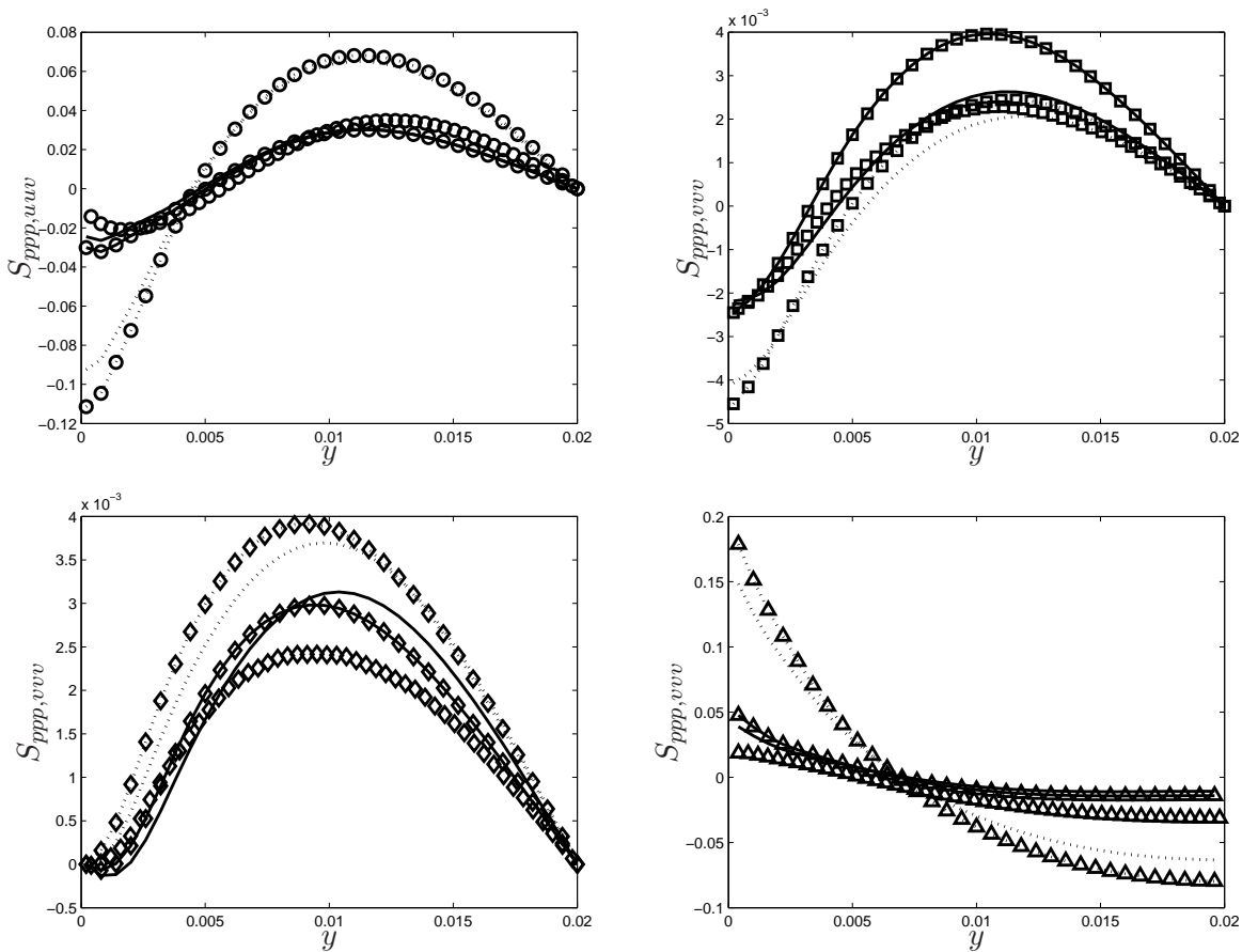
FIG. 6.6 – Comparaison des corrélations triples prédites par les différents modèles pour le cas B3. \circ : lagrangien stochastique ; — : équation (6.14) ; — \circ — : équation (6.14) avec correction (6.18) ; \dots\dots : équation (6.16) ; \dots\dots\circ\dots\dots : équation (6.16) avec correction (6.18).
