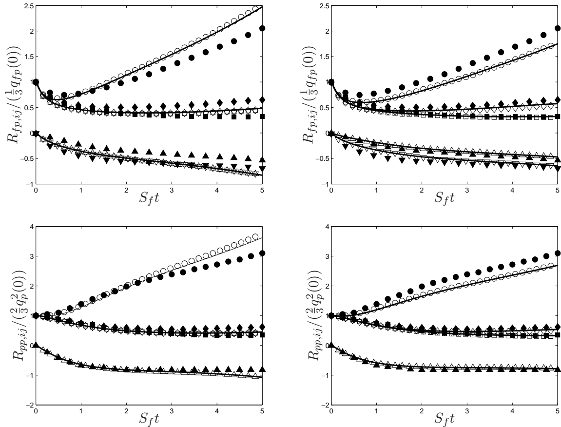
FIG. 5.11 – Développements des contraintes cinétiques (cas B) prédits par le modèle SLM (gauche) et le modèle NCLIPM (droite). \circ : lagrangien stochastique ; — : eulérien ; \bullet : LES/DPS (Laviéville [1997]).
