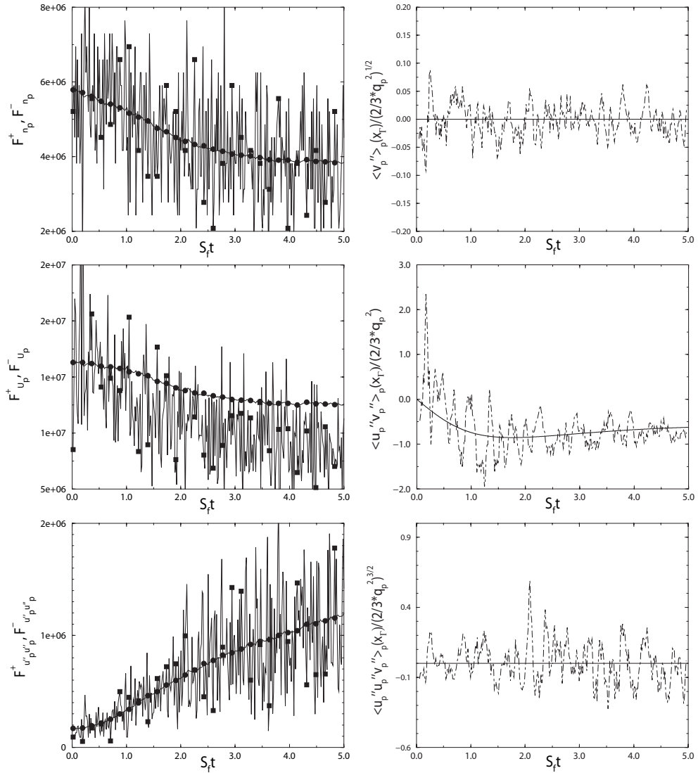
FIG. 5.24 – Développements des flux de n_p , U_p et R_{pp,uu} . gauche : demi-flux entrant ( \circ ) et demi-flux sortant ( \square ). droite : condition de flux imposée au domaine eulérien associée aux demi-flux de gauche et moyennée sur \Delta t = \delta dt_{eul} ( \dots\dots ) et valeurs théoriques ( \text{—} ).
