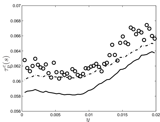
FIG. 2.3 – Comparaison des prédictions a priori du temps caractéristique de collision avec les temps mesuré par une simulation lagrangienne stochastique dans le cas du canal du chapitre 6. \circ : mesures dans la simulation lagrangienne stochastique ; — : modèle isotrope ; - · - · - : modèle anisotrope.
