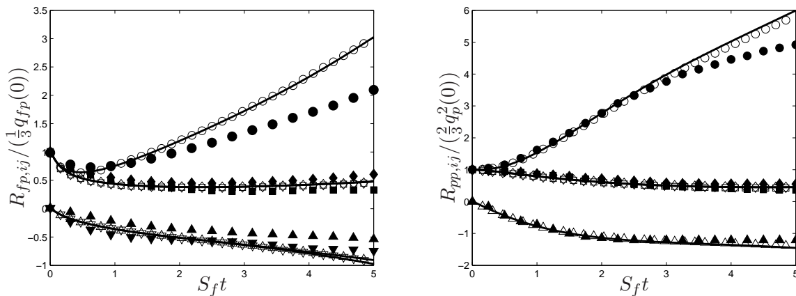
FIG. 5.25 – Développements des contraintes fluide-particules (gauche) et des contraintes particulaires (droite) prédites par HELM avec \eta = 0,3 . \circ : moyenne dans le domaine lagrangien ( \circ : R_{uu} , \square : R_{vv} , \diamond : R_{ww} , \triangle : R_{uw} ) ; — : moments au centre du domaine eulérien ; \bullet : LES/DPS (Laviéville [1997]).
