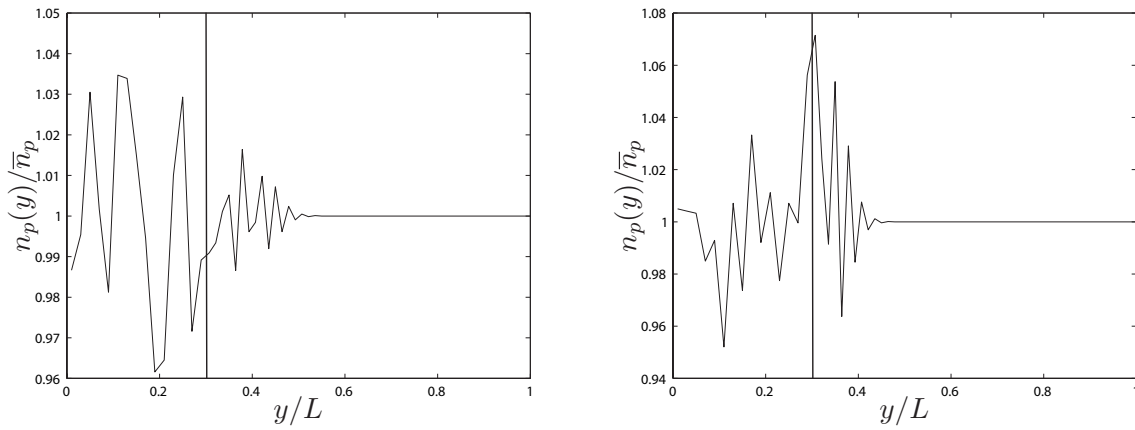
FIG. 5.35 – Profils de densité de particules à l’instant t = 5/S_f issus de HELM avec \eta = 0, 3 pour le cas B (gauche) et la cas Ac (droite).
