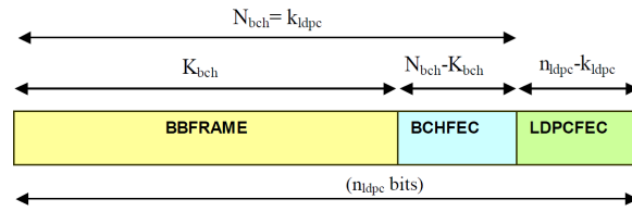
FIGURE 5.3 – Format des données avant entrelacement de bits
