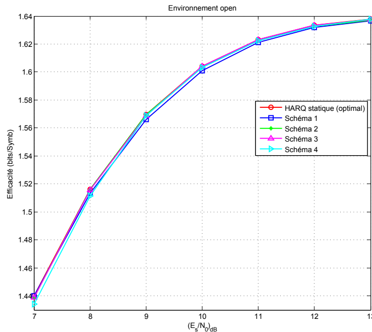
FIGURE 3.15 – Comparaison de l'efficacité obtenue dans l'environnement open avec le cas optimal et les différents schémas considérés pour différentes valeurs de E_s/N_0 .
