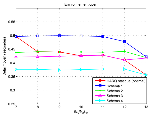
FIGURE 3.17 – Comparaison de délais obtenus dans l'environnement open avec le cas optimal et les différents schémas considérés pour différentes valeurs de E_s/N_0 .
