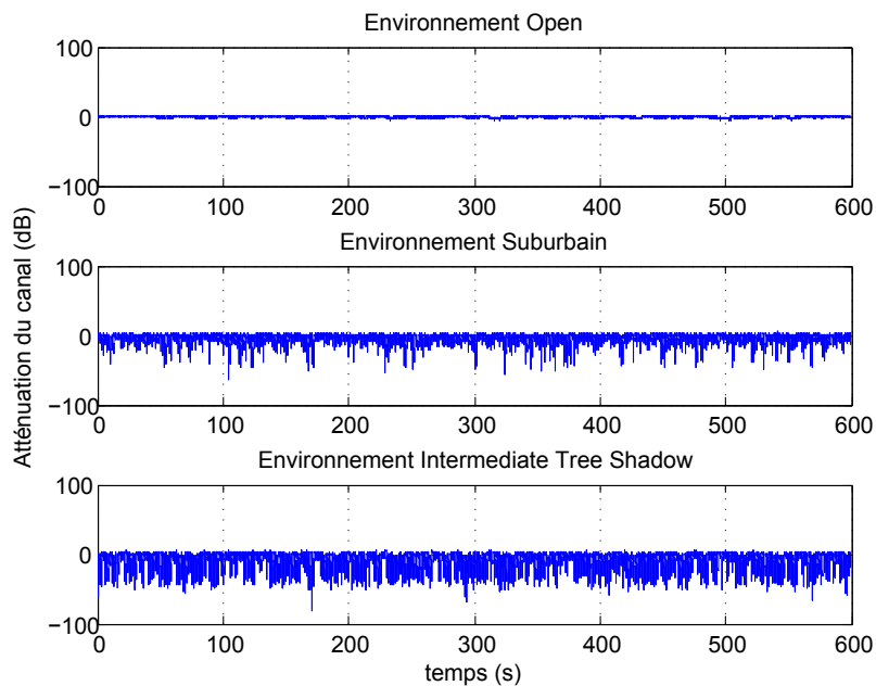
FIGURE 3.1 – Traces du canal LMS en bande S pour différents types d'environnement avec une vitesse de terminal mobile 60 Km/h
