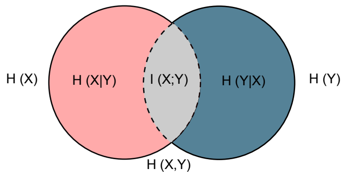
FIGURE 2.8 – Diagramme de Venn pour diverses mesures d'information liées à des variables corrélées X et Y .
