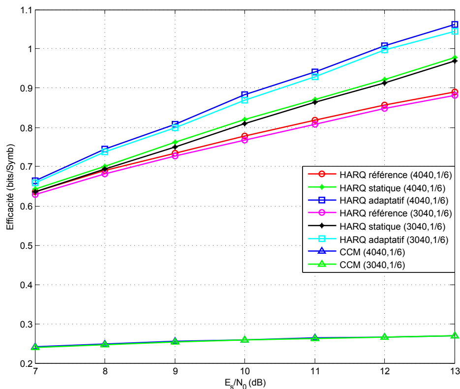
FIGURE 5.15 – Efficacité obtenue avec les méthodes considérées en utilisant les codes (4040,1/6) et (3040,1/6), et trames à petite taille, pour des messages IP de taille 1500 octets
