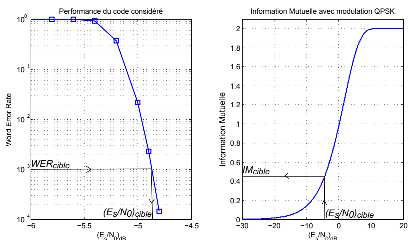
FIGURE 3.5 – Exemple de calcul de IM_{cible} en utilisant la courbe de performance du code considéré et la courbe de l'information mutuelle (modulation QPSK).
