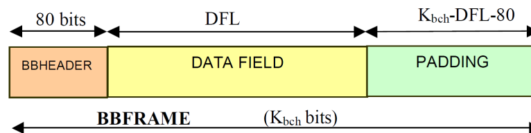
FIGURE 5.2 – Format de BBFRAME à la sortie de l’adaptateur de flux
