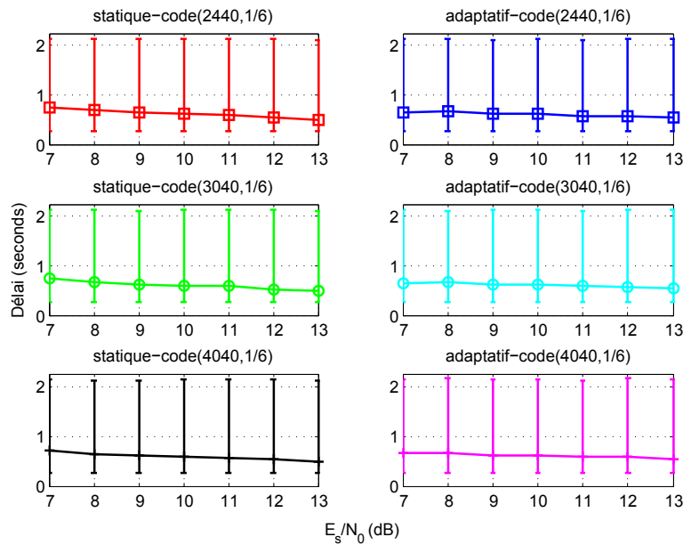
FIGURE 5.14 – Délais moyens, minimaux et maximaux obtenus avec les deux méthodes adaptative et statique pour différents codes considérés et leurs tailles de trame correspondants, pour des messages IP de taille 1500 octets.
