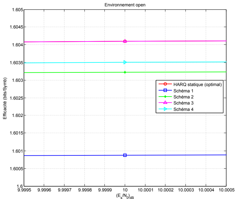
FIGURE 3.16 – Zoom sur les différentes courbes d'efficacité obtenues pour une valeur de E_s/N_0 = 10dB .
