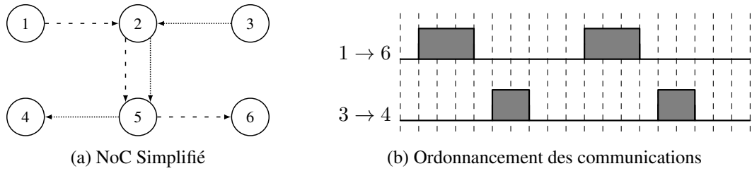
Figure A.7: Exemple d'application de la règle 2 du modèle d'exécution avec 2 communications partageant un lien NoC ② → ⑤
